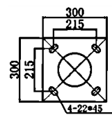
DISTANCIA ENTRE PERNOS PARA ALTURAS: 3M-3,5M-4M-5M-6MTS.
