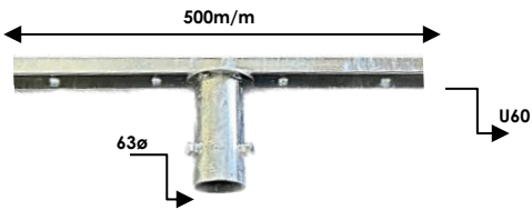
CRUCETA 1 PROYECTOR
