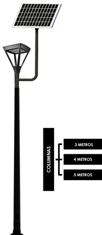
Conjunto 1: Columna Troncoconica 3mts, 4mts Y 5mts Con Luminaria DELTA T-70N Solar LED
