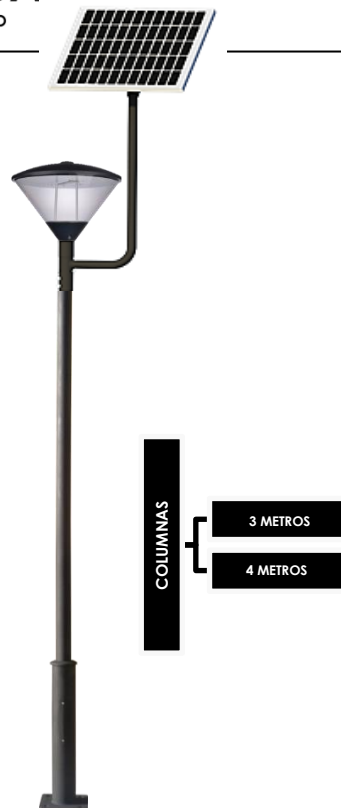
Conjunto 2: Columna OPORTO 3mts, 4mts Con DIABOLO FUTURE T-020A Solar LED
