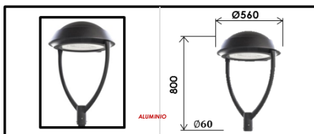
ECA INVERTIDA D-32L LED SOLAR CREE XTE 45W-7200LM
