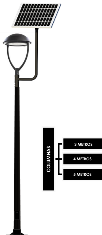
Conjunto 1: Columna Troncoconica 3mts, 4mts Y 5mts Con ECA INVERTIDA D-32L Solar LED
