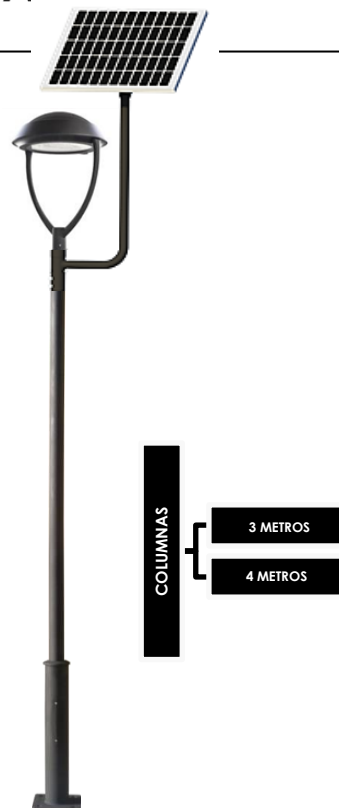
Conjunto 2: Columna OPORTO 3mts, 4mts Con ECA INVERTIDA D-32L Solar LED
