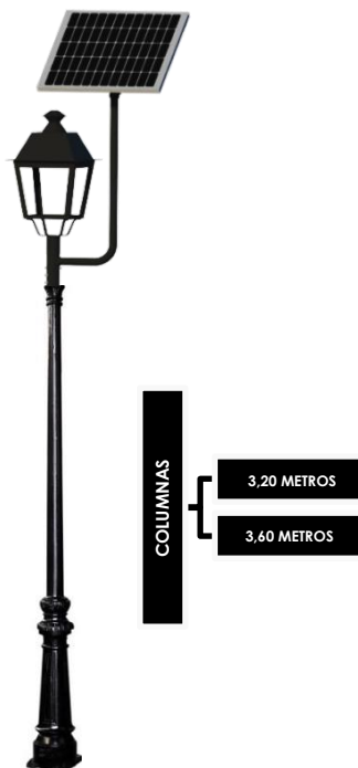
Conjunto 3: Columna Villa 3,20mts -3,60mts Con FAROL VILLA SOLAR LED
