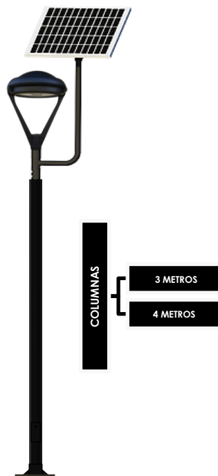
Conjunto 3: Columna Cilindrica 3mts, 4mts Con LUM.PREMIUM T-20L Solar LED
