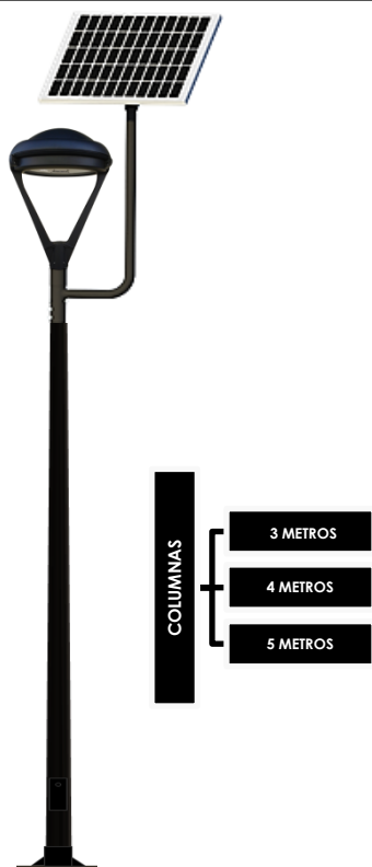
Conjunto 1: Columna Troncoconica 3mts, 4mts Y 5mts Con LUM.PREMIUM T-20L Solar LED
