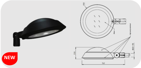
COMO OPCIONAL GRABADO LASER ESCUDO CIUDAD BRAZO PARED MOD. CADIZ RAL 9005 NEGRO MATE. FIJACION CENITAL/SUSPENDIDO
