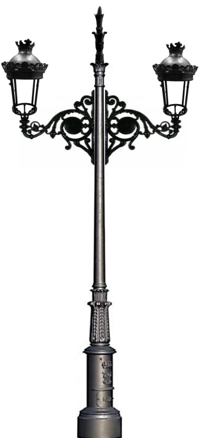
Conjunto 2: Columna Fernandina/Bailen 4,15mts Con 2 Brazos Fernandino+ 2 Farol Ecofernandino LED Y Remate Superior Tipo Lanza 70Cm
