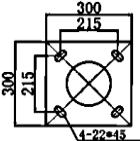
DISTANCIA ENTRE PERNOS PARA ALTURAS: 3M-3,5M-4M-5M-6MTS.
