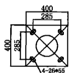
DISTANCIA ENTRE PERNOS PARA ALTURAS: 7MTS-8MTS.
