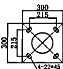
DISTANCIA ENTRE PERNOS
