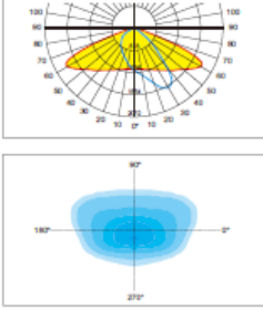
OPTICA ABT-130°X136°
