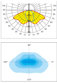
OPTICA ABP-75°X135°
