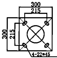
COLUMNA DOBLE TR2-T-20L VERUS AROS BLACK
