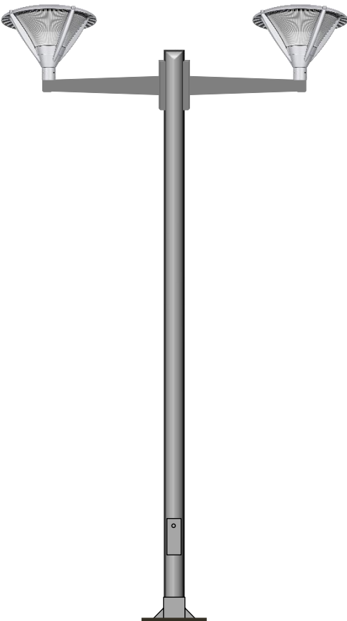
Conjunto 2:Columna Troncoconica Con 2 Brazos Premiun+2 Lum. T-050
